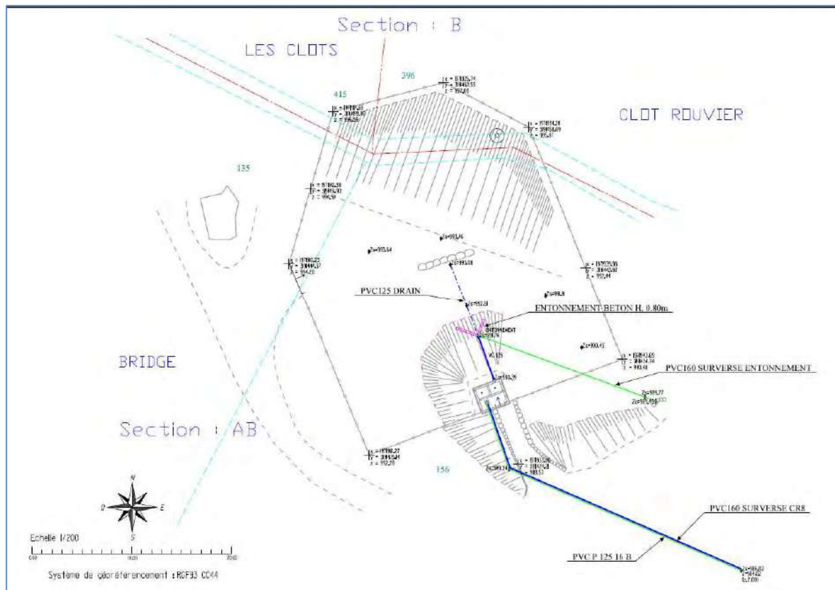
Figure 2 : Plan de situation sur plan parcellaire (extrait du plan conforme à exécution de Maurel TP)
