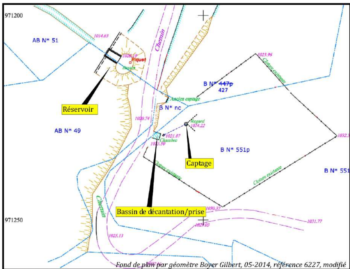
Figure 2 : Plan de situation sur plan parcellaire
