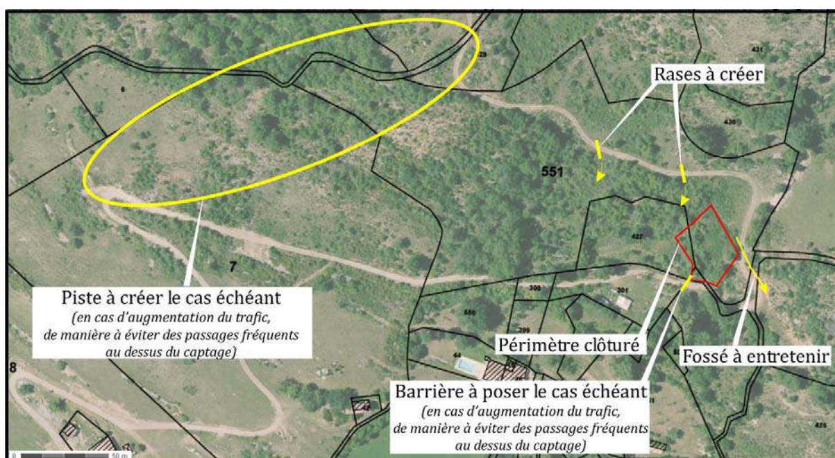
Figure 4 : Aménagements des abords du captage
