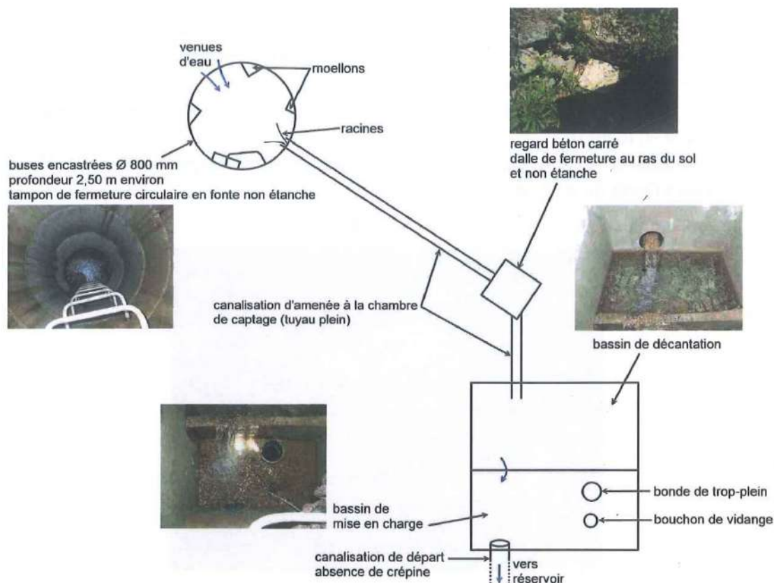
Figure 3 : Schéma du captage des Ferrayes (d'après Téhtys Hydro, 2013)
