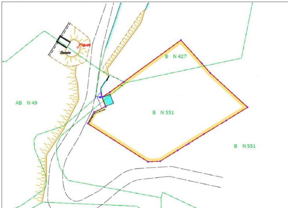
Figure 22: Plan du PPI du captage des Ferrayes (source : Boyer, Géomètre Expert)
