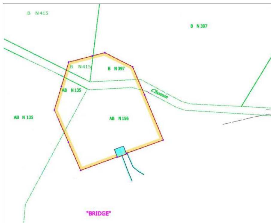
Figure 21: Plan du PPI du captage de Briges (source : Boyer, Géomètre Expert)
