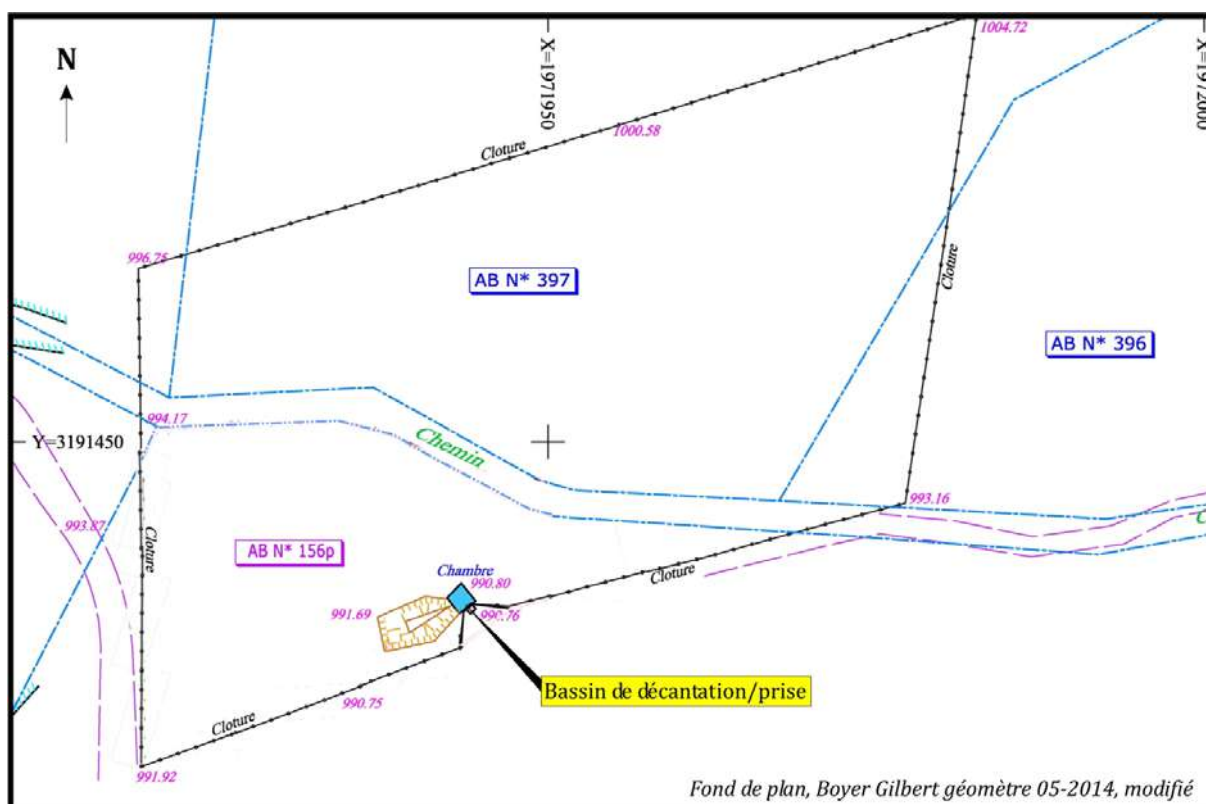
Figure 2 : Plan de situation sur plan parcellaire
