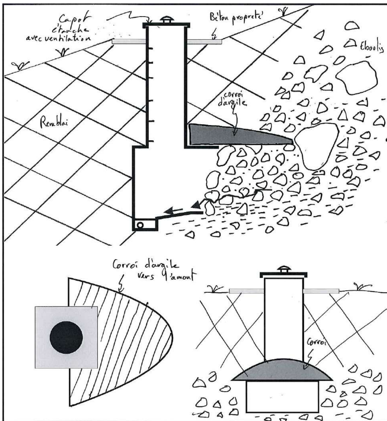
Principe de recaptage
