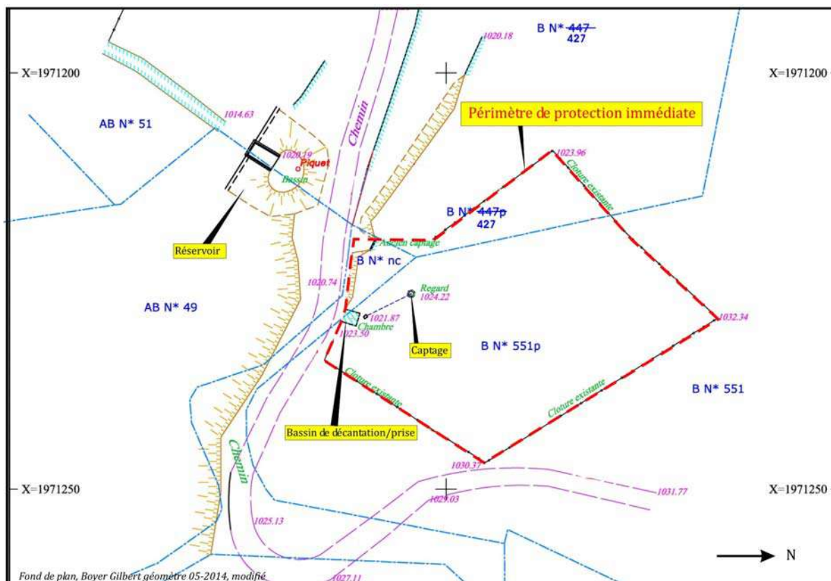
Figure 5 : Périmètre de protection immédiate de la source des Ferrayes
