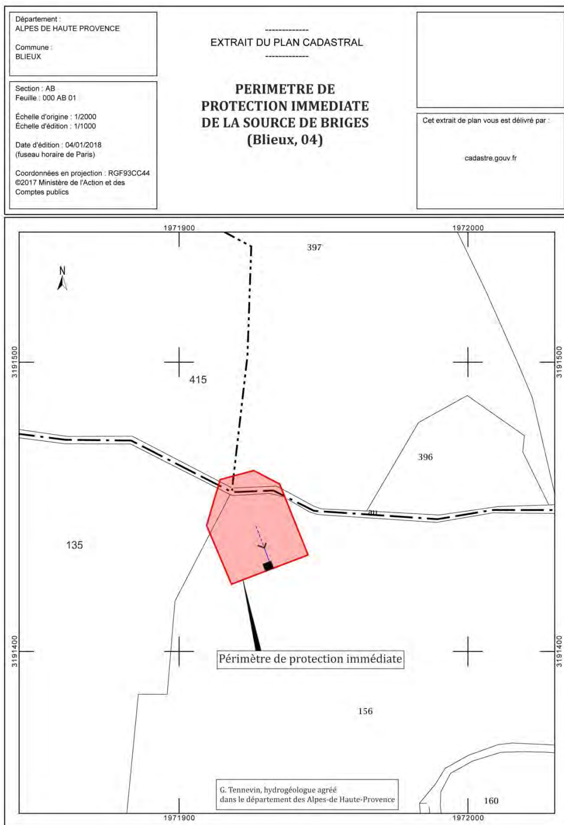
Figure 4 : Périmètre de protection immédiate de la source de Briges
