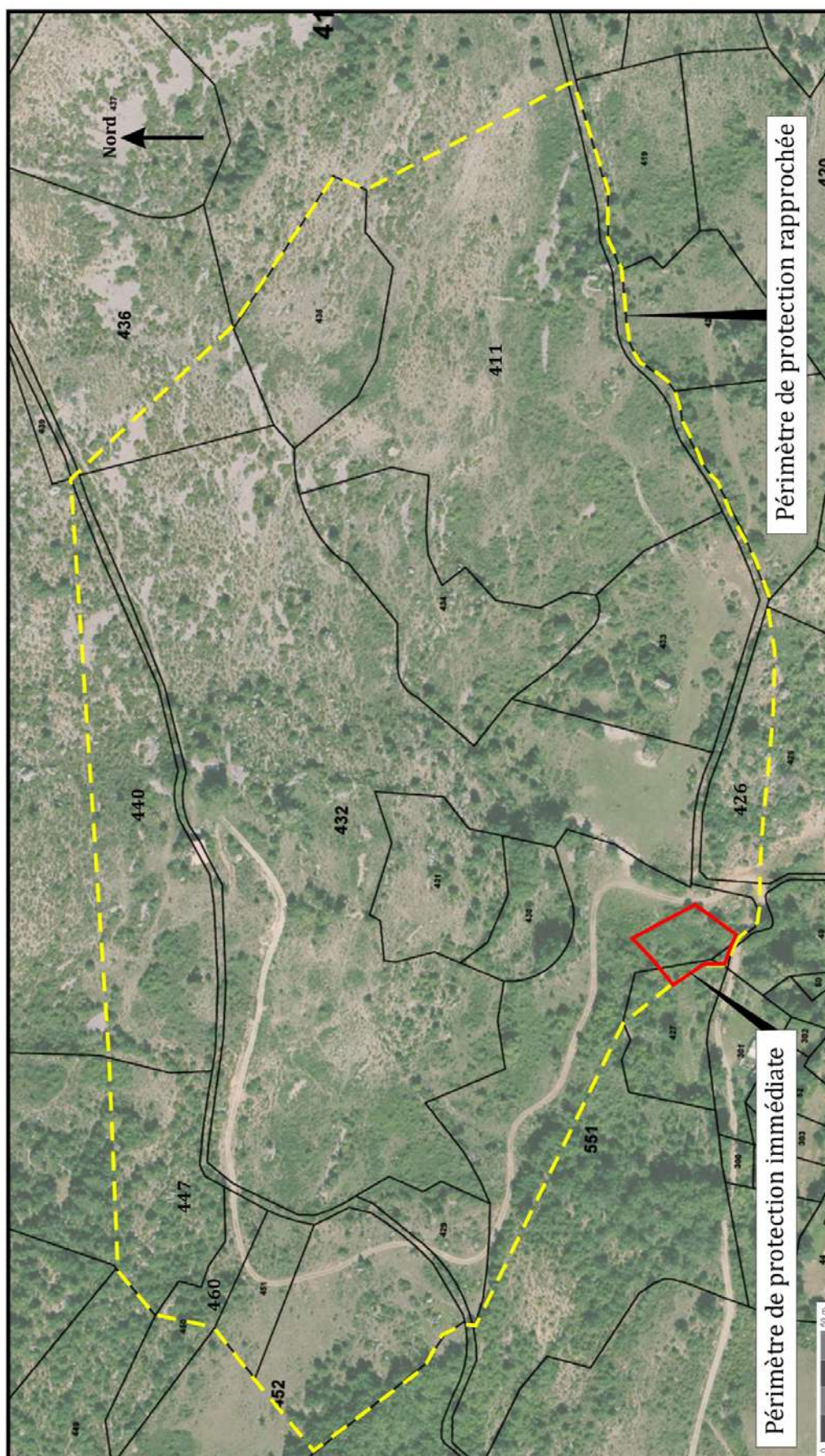
Figure 6 : Périmètre de protection immédiate et rapprochée de la source des Ferrayes
