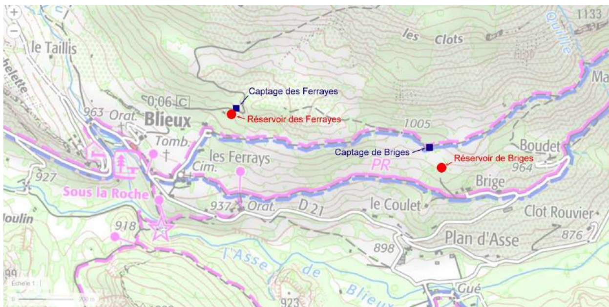
Figure 5: Situation des réservoirs de Ferrayes et de Briges (source : géoportail.gouv)
