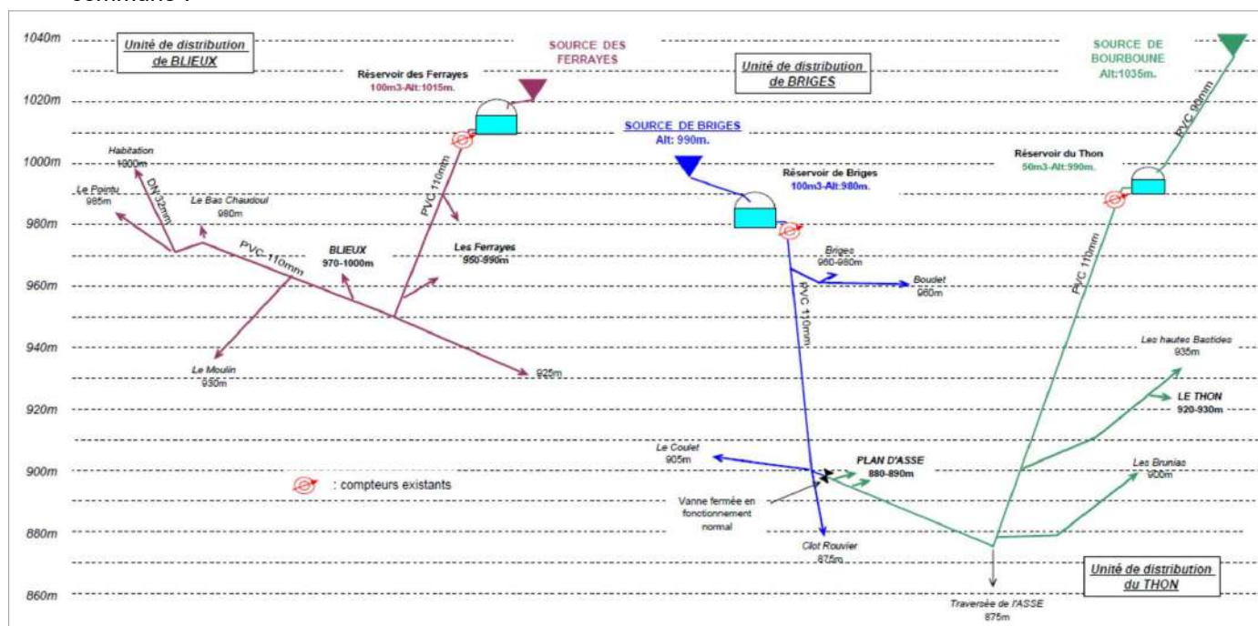
Figure 4: Schéma synoptique du réseau AEP de Blieux
