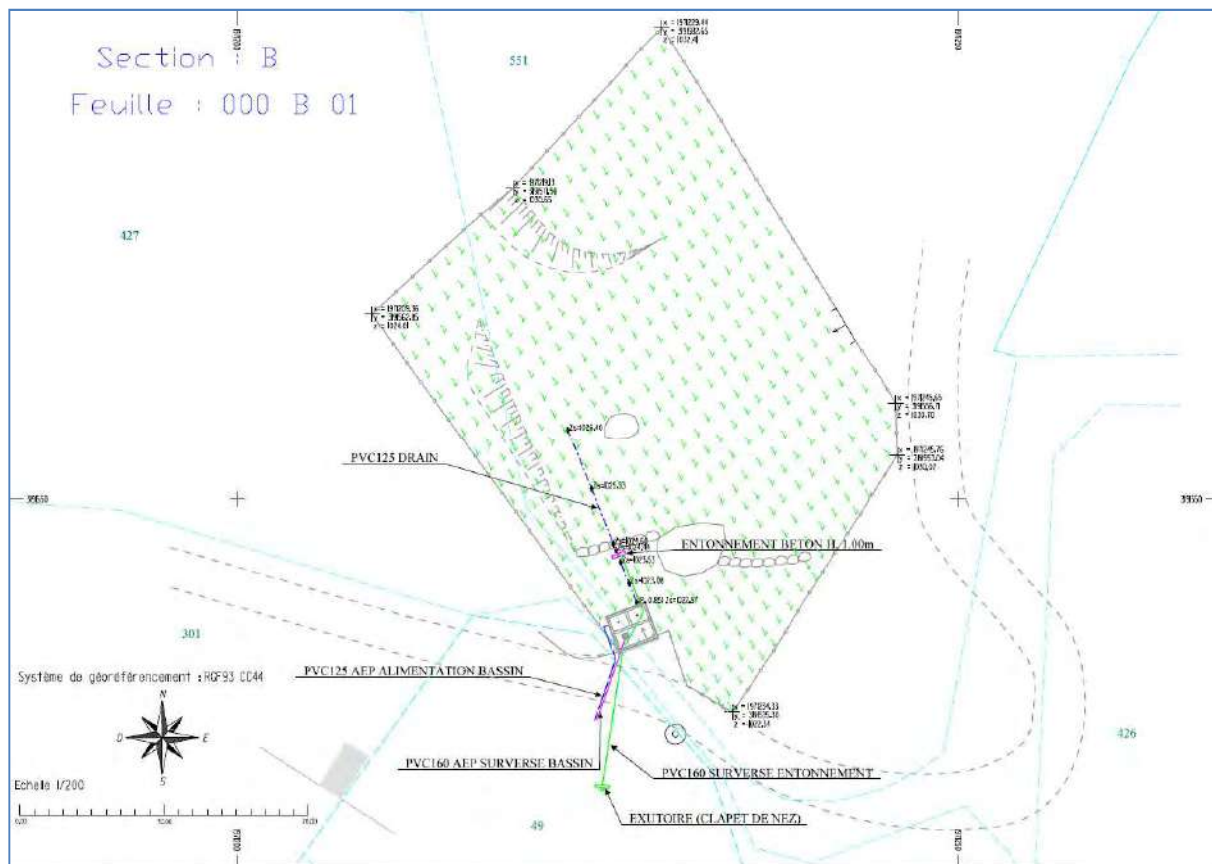
Figure 2 : Plan de situation sur plan parcellaire
