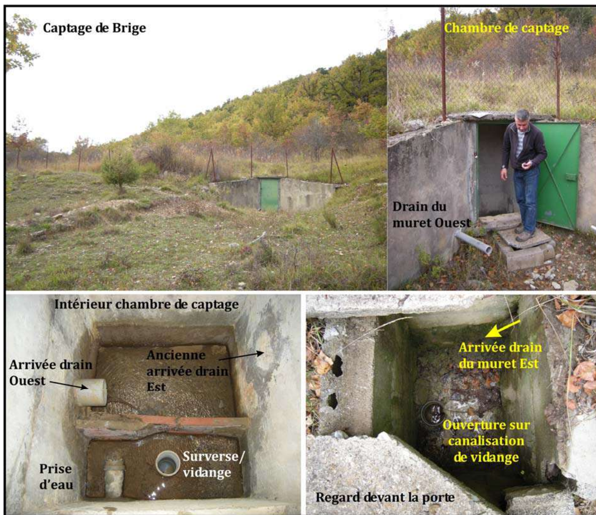
Figure 3 : Captage de la source de Brige
